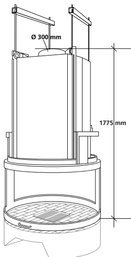
Vue perspective foyer ouvert
