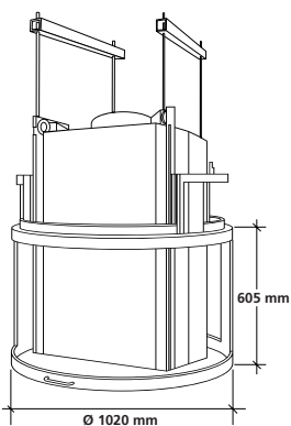
Vue perspective foyer ouvert
