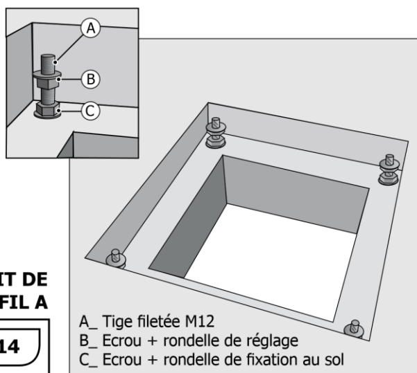
A_ Cadre inox à retirer B_ Ecrous pour retirer le cadre (x12) C_ Réservation D_ Trous à percer pour tige filetées (x4)
