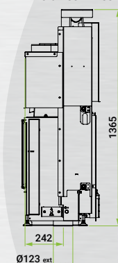
VERSION SURBAISSÉE
